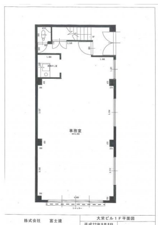
大栄ビル 1階平面図 現況優先
